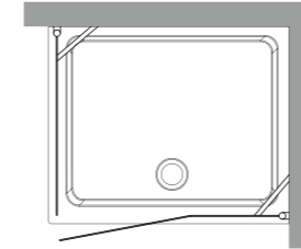
9142 Cabina doccia SX con porta battente in linea e fisso laterale per piatto doccia 80x96 SX apertura lato 96. Apertura utile 54 cm, altezza 180 cm. Left shower enclosure with door for left shower-tray 80x96 opening on 96 side. Usable opening 54 cm, height 180 cm.
