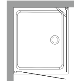
9144 Cabina doccia DX con porta battente e fisso laterale per piatto doccia 80x96 SX apertura lato 80. Apertura utile 65 cm, altezza 180 cm. Right shower enclosure with door for left shower-tray 80x96 opening on 80 side. Usable opening 65 cm, height 180 cm.
