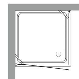
9160 Cabina doccia DX con porta battente e fisso laterale per piatto doccia angolare 80x80 quadro. Apertura utile 72 cm, altezza 180 cm. Right shower enclosure with door for corner shower-tray 80x80. Usable opening 72 cm, height 180 cm.
