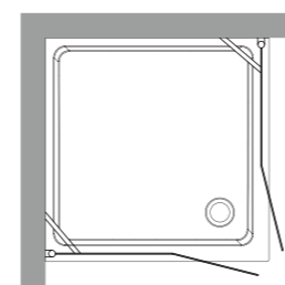
9145 Cabina doccia DX/SX a due porte battenti e fisso in linea per piatto doccia 90x90 quadro. Apertura utile 36 cm più anta, altezza 180 cm. Reversible shower enclosure with two door for corner shower-tray 90x90. Usable opening 36 cm each door, height 180 cm.
