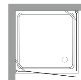
9146 Cabina doccia DX con porta battente e fisso laterale per piatto doccia angolare 90x90 quadro. Apertura utile 72 cm, altezza 180 cm. Right shower enclosure with door for corner shower-tray 90x90. Usable opening 72 cm, height 180 cm.
