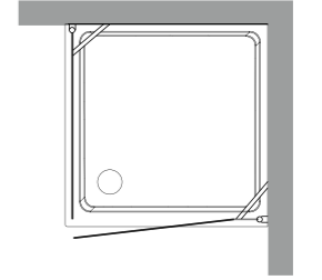
9161 Cabina doccia SX con porta battente e fisso laterale per piatto doccia angolare 80x80 quadro. Apertura utile 72 cm, altezza 180 cm. Left shower enclosure with door for corner shower-tray 80x80. Usable opening 72 cm, height 180 cm.
