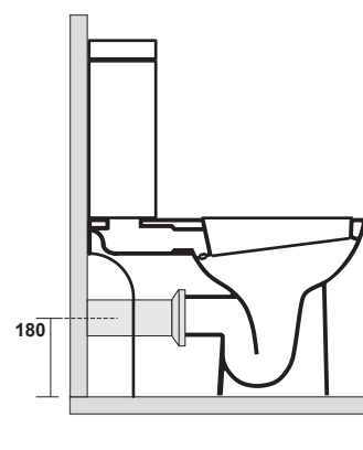
raccordo di scarico a parete art. 7539 connector for wall outlet art. 7539
